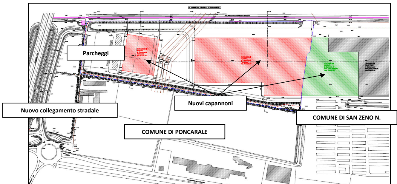
Figura 1 – Planimetria generale di progetto
